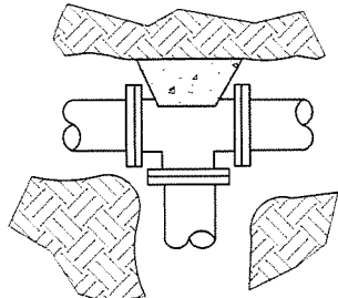
TEE
